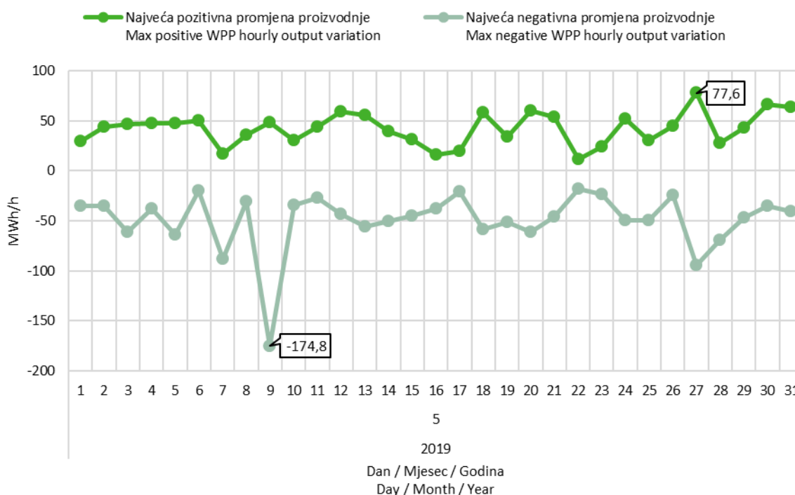
Slika 9 Maksimalna pozitivna i maksimalna negativna promjena satne proizvodnje VE u svibnju 2019. godine
