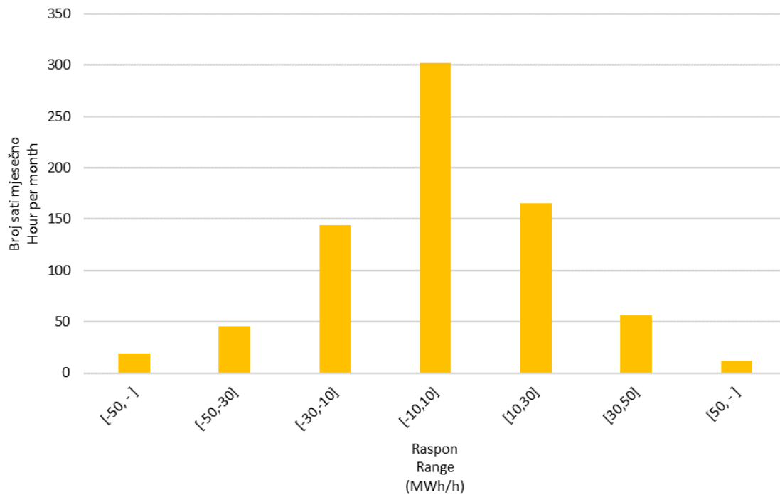
Slika 10 Statistička raspodjela satnih promjena proizvodnje VE u svibnju 2019. godine
