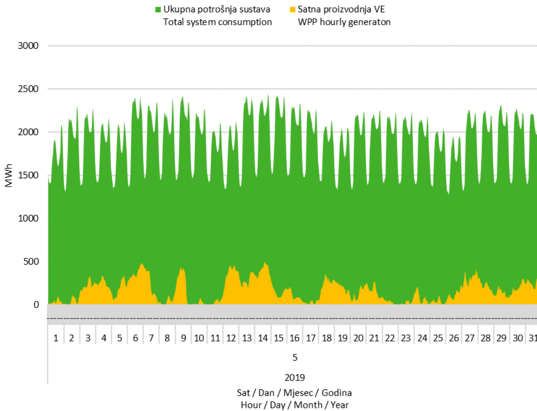
Slika 7 Usporedba satnog dijagrama opterećenja sustava i proizvodnje vjetroelektrana u svibnju 2019. godine
