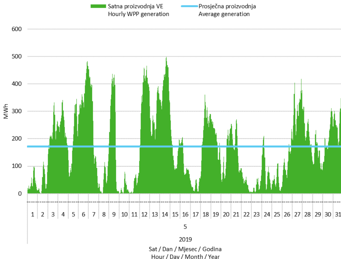
Slika 2 Satna proizvodnja svih vjetroelektrana u svibnju 2019. godine
