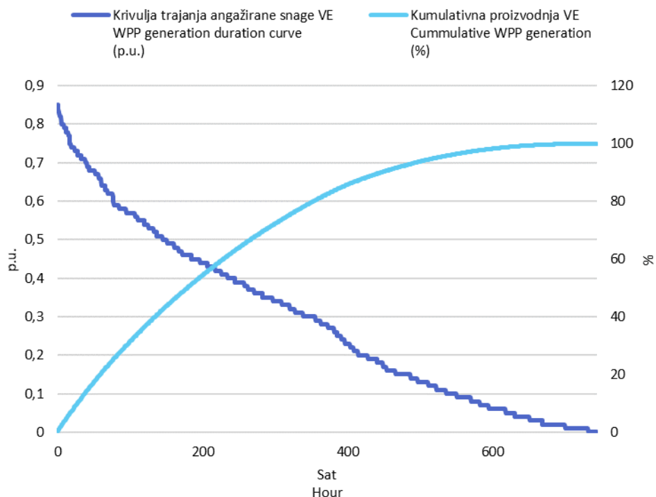
Slika 3 Krivulja trajanja angažirane snage svih VE i kumulativna proizvodnja VE u svibnju 2019. godine u jediničnim vrijednostima
