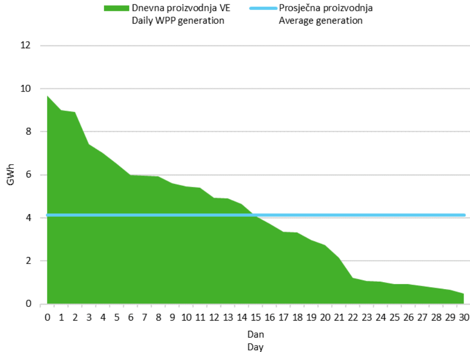
Slika 6 Krivulja trajanja dnevne proizvodnje vjetroelektrana u svibnju 2019. godine
