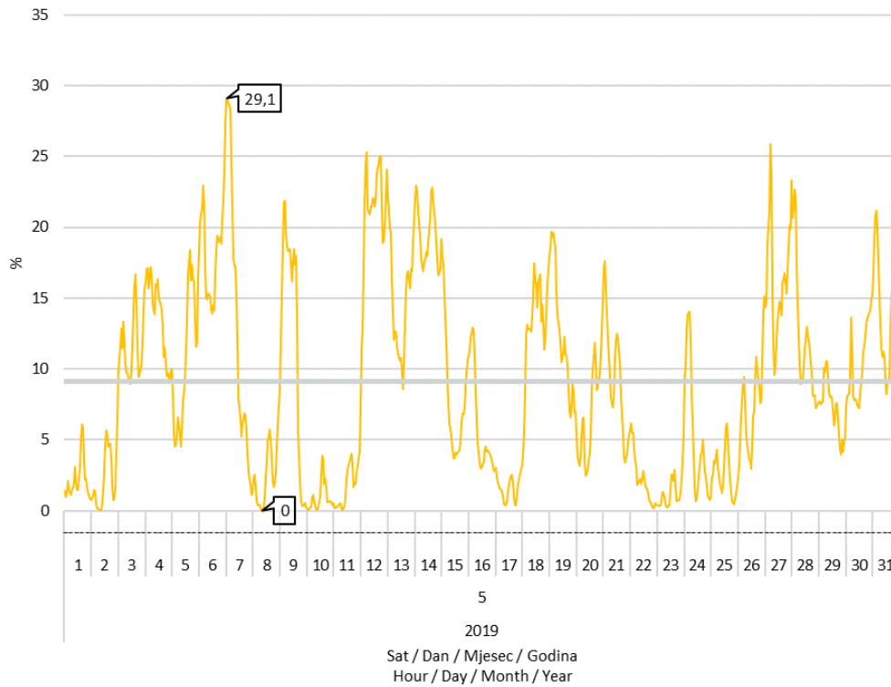
Slika 8 Udio proizvodnje vjetroelektrana u pokrivanju satnog opterećenja elektroenergetskog sustava u svibnju 2019. godine
