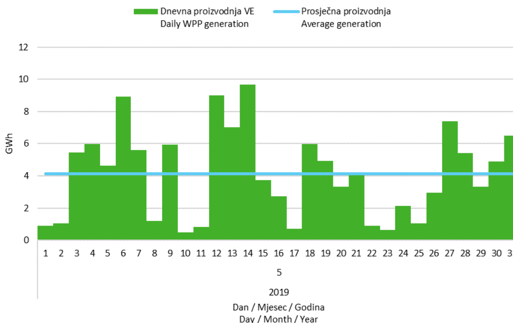
Slika 5 Dnevna proizvodnja svih vjetroelektrana u svibnju 2019. godine
